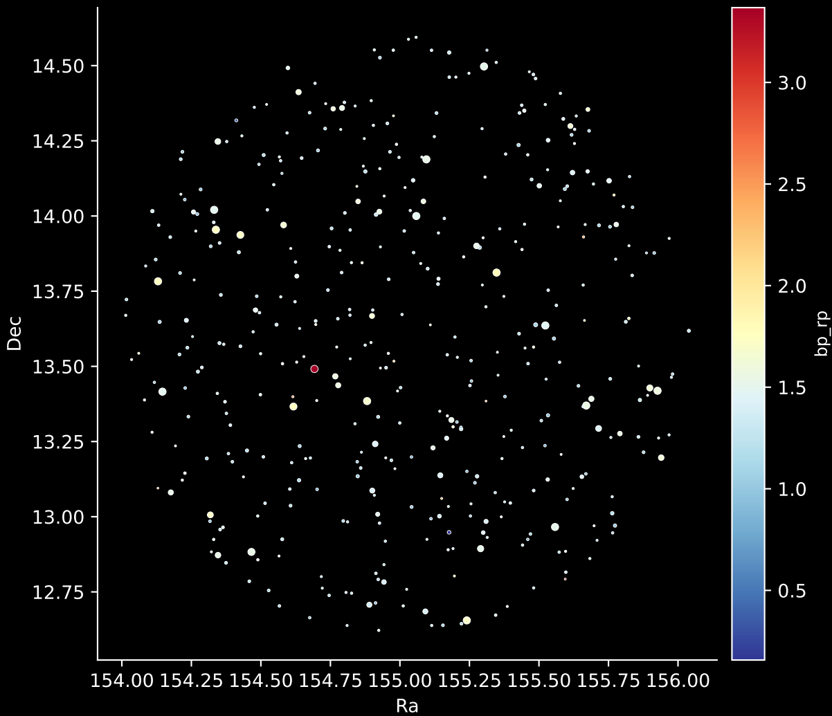
GALAH DR4 Field: [6600] Stars: 423
