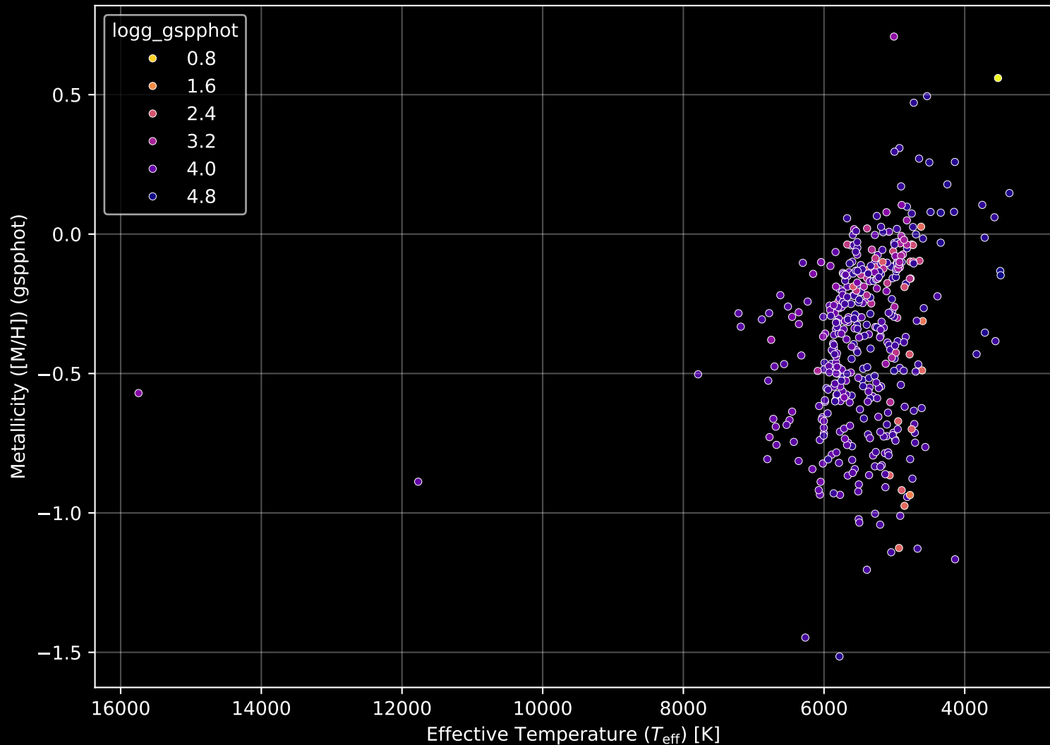
GALAH DR4 Field: [6600] Stellar Population Parameters (n= 423)
