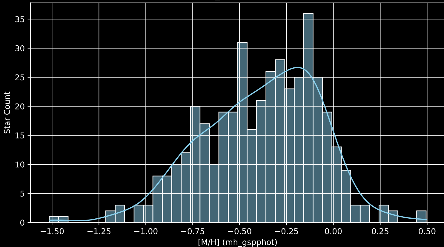
GALAH DR4 Field: [6600] [M/H] (mh_gspphot) (n= 421)
