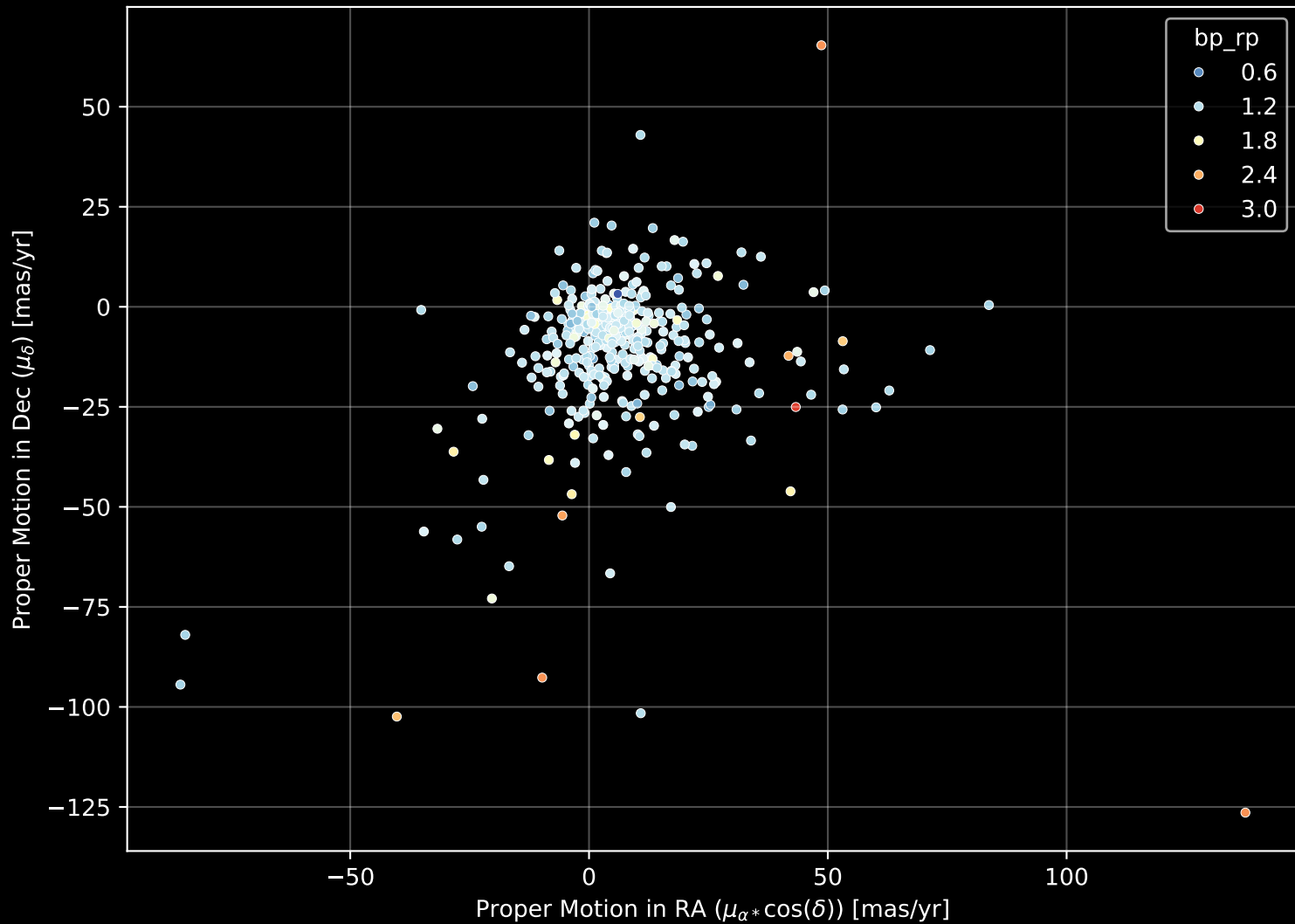
GALAH DR4 Field: [6600] Proper Motion Diagram (n= 423)
