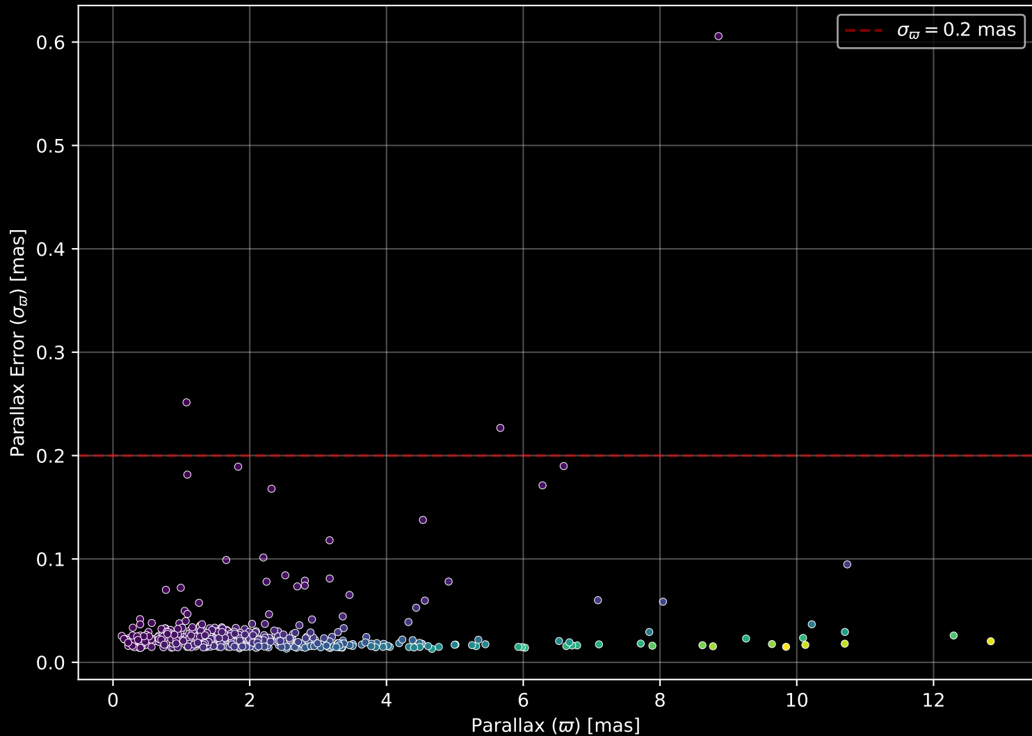
GALAH DR4 Field: [6600] Parallax Quality (n= 423)
